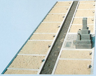
卷石施工例
